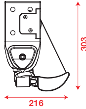
inclinazione massima 85°
